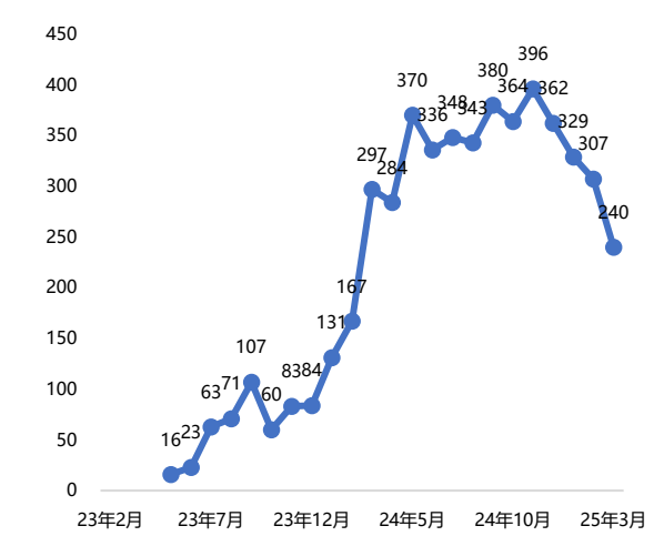
1 智谱清言
