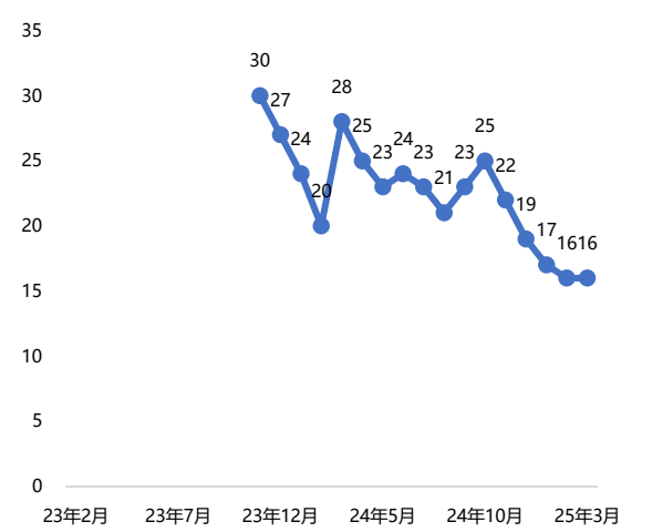
10 万兴PDF
